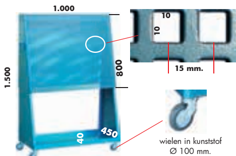
Geperforeerd paneel met rubberwielen.
