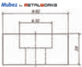
Mubea matrijsreductie MBN50606-2.
