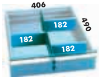
laden geleverd met 1 scheidingswand en 3 tussenschotten (behalve 300mm)
