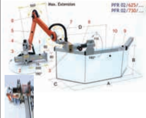
Veiligheidsafscherming voor universele freesmachines.
