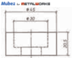
Mubea matrijsreductie MBN50606-1.
