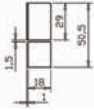
Voor ML 720 tot 1920mm Totale lengte is ML + 166mm Installatie lengte is ML + 132mm
